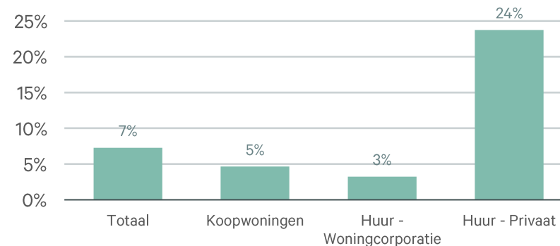
Ontwikkeling woningvoorraad (2015-2020)
